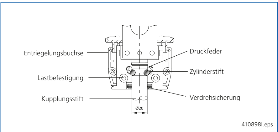
Die Schnellwechselkupplung am Steuergerät DSM-C
