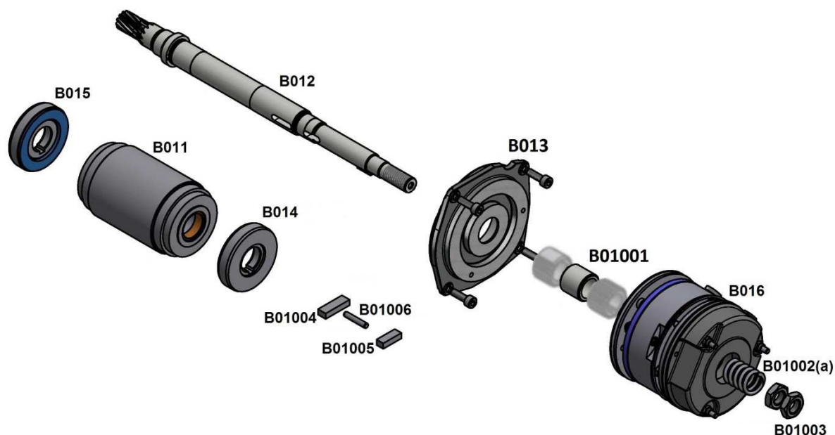
Einfachbremse
